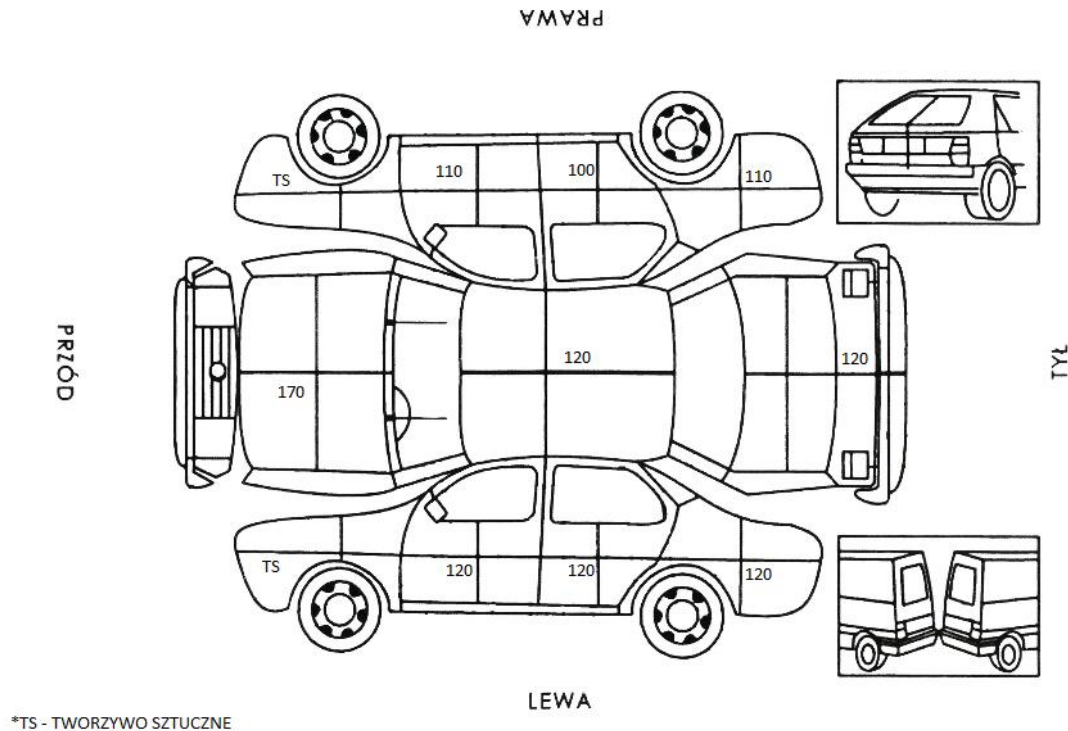
Rys.6. Pomiar powłoki lakierniczej na pojeździe
